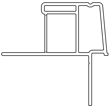
#4598 Fermé Moulure 1"
